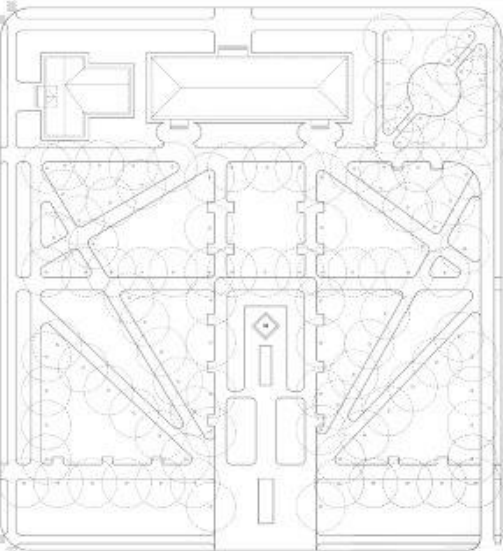
ПЛАН РАССТАНОВКИ ОСВЕТИТЕЛЬНЫХ ПРИБОРОВ
