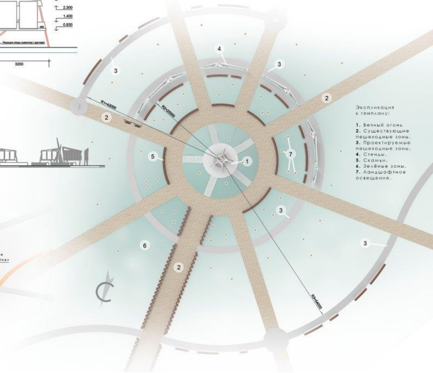
Генплан
