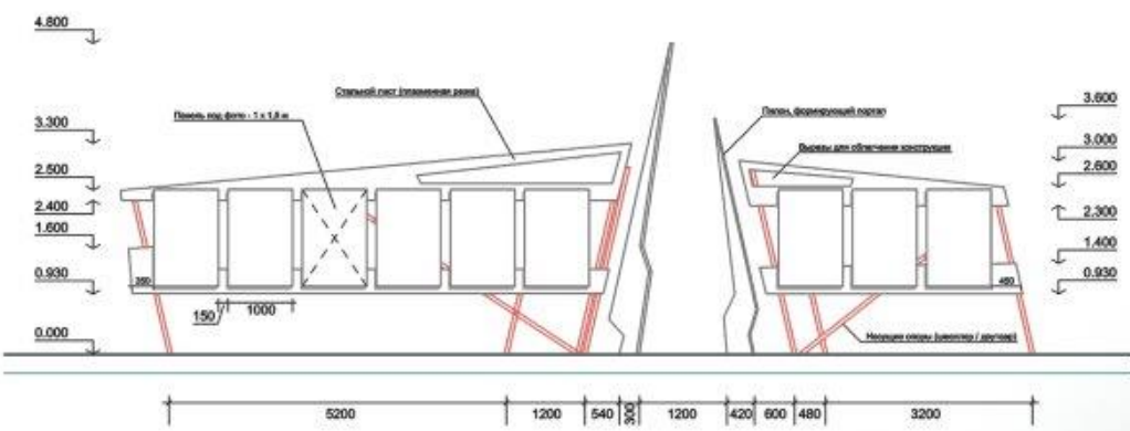
Фасад стены
